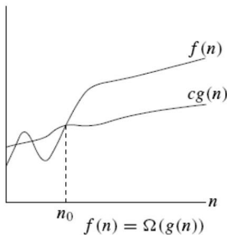
Gambar 2 Kurva f(n) akan selalu berada diatas cg(n) pada n \geq n_0 .
