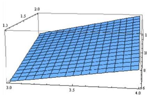
Gambar 4 Output pada interval x = \{x | 1 \leq x \leq 2\} .
