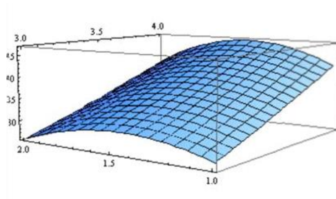
Gambar 1 Output pada interval x = \{x|3 \leq x \leq 4\}; t = \{t|1 \leq t \leq 2\} .
